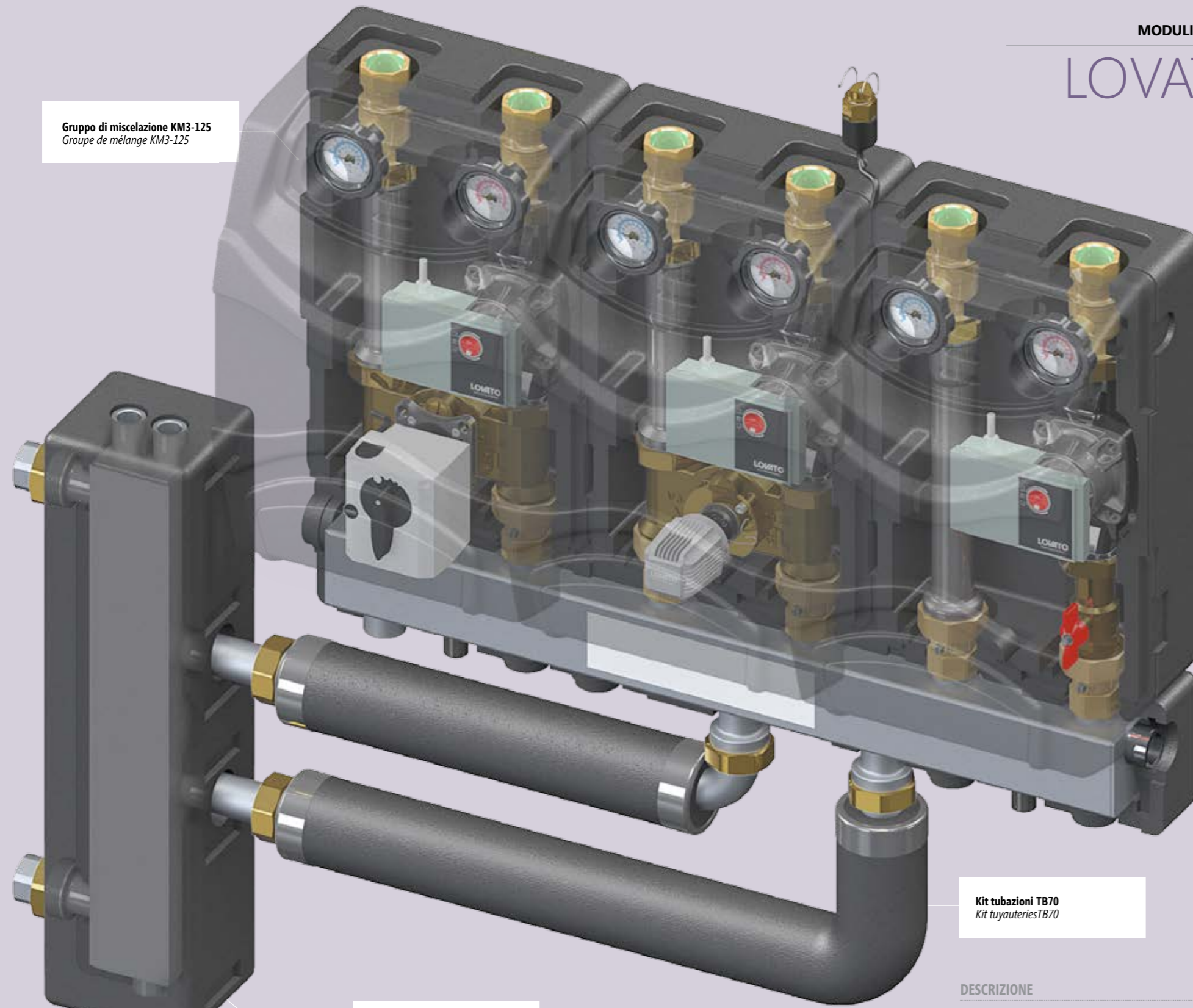
Separatore idraulico CP70 Séparateur hydraulique CP70
