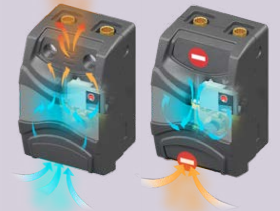
Gruppo di miscelazione KTC-125 Groupe de mélange KTC-125
